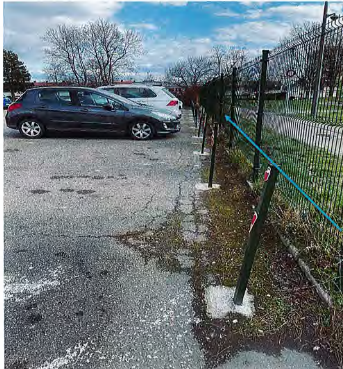
POSE DE 3 PEHD Ø40 + 1 L1T FREE Tranchée traditionnelle sur terrain naturel Remblai avec extraît - Réfection en ENROBE
